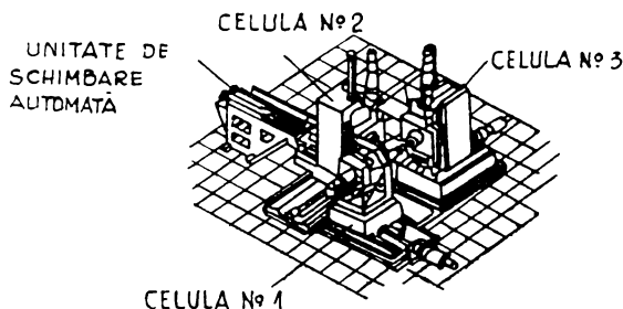
Fig. 6. Complex de uzinare.
