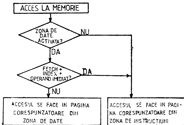
Fig.3-3 SELECTIA ZONEI DE INSTRUCIUNI SAU DE DATE
