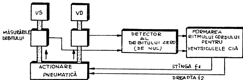
Figura 14. Schema-bloc a sistemului de reglare totală a inimii artificiale folosind mecanismul Frank-Starling: VS — ventricolul stâng, VD — ventricolul drept al CIA.
